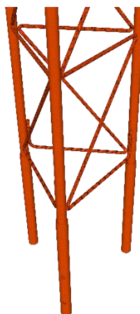
Vista inferior sección de torre
