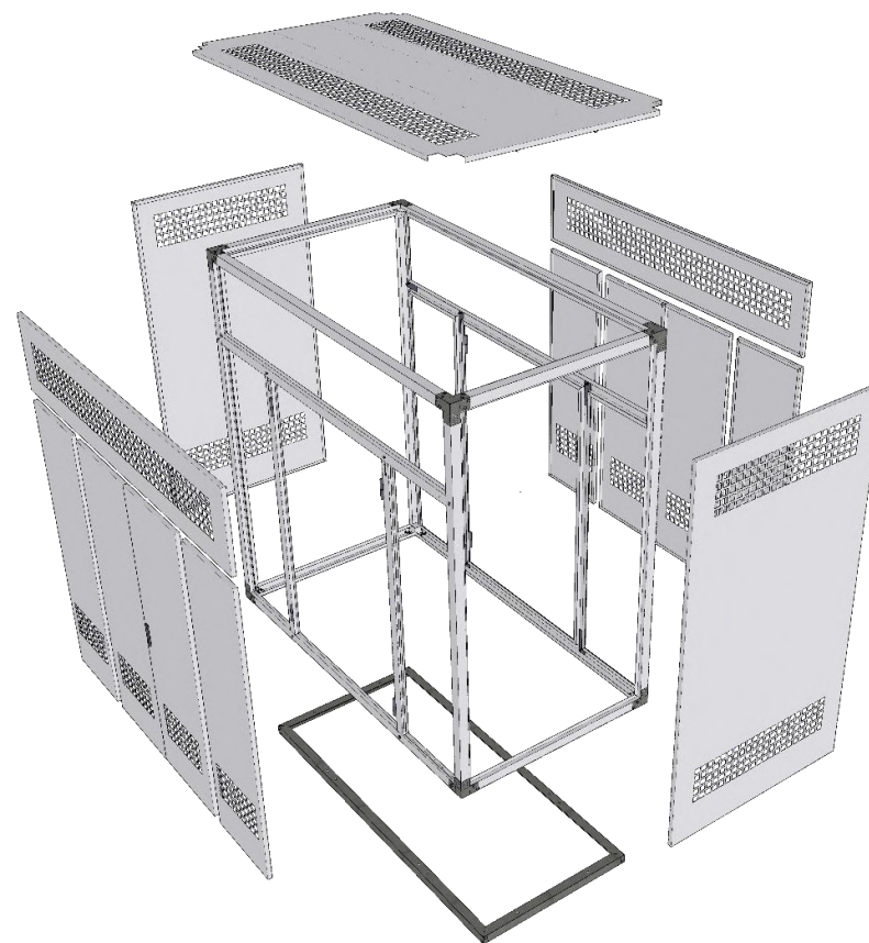
Gabinete desarmado
